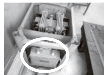
電気溶接機の側面に取り付けられた 低圧コンデンサー
