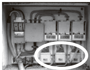
低圧分電盤内の低圧コンデンサー
